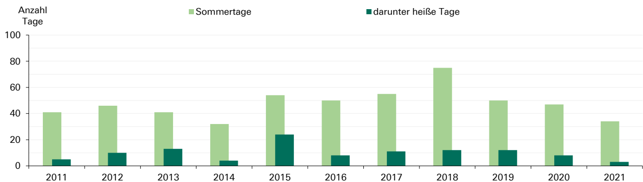
Abb. 3: Sommertage und heiße Tage
