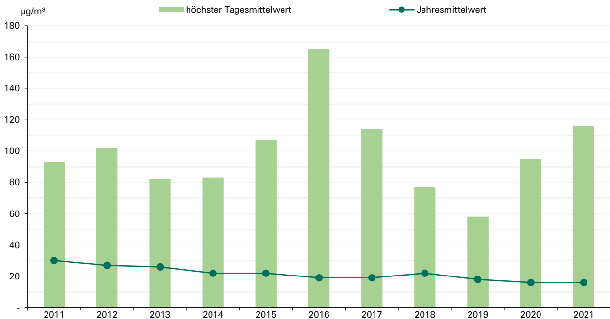
Abb. 7: Feinstaubkonzentration (PM 10 ) an der Messstation Königsplatz
