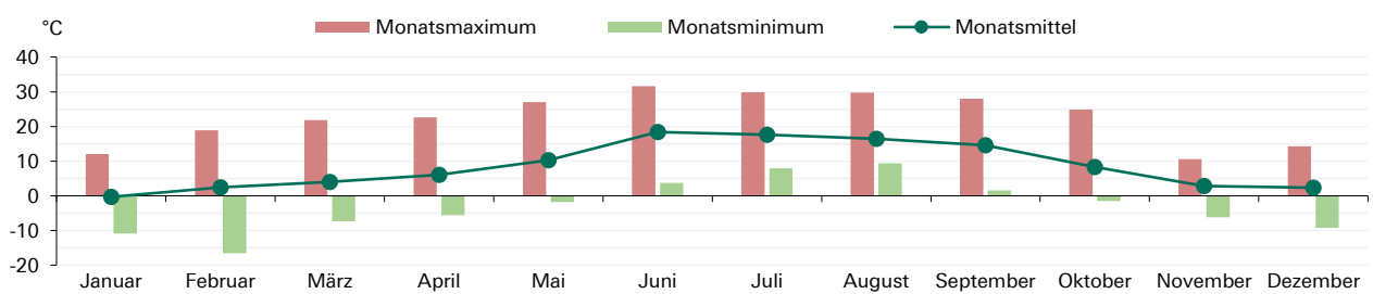
Abb. 2: Lufttemperatur - Extremwerte und Monatsmittel nach Monaten (2021)
